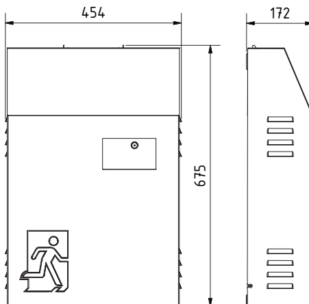
Abb. 4: Maßzeichnung LPS 230-500-S
