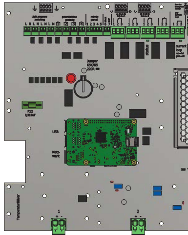
Abb. 30: USB-Anschlüsse an der Hauptplatine
