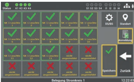
Abb. 93: Maske „Leuchten Daten – Leuchten hinzufügen“
