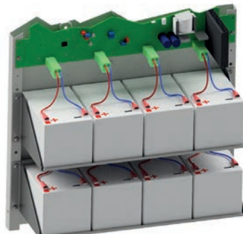
Abb. 13: Batterieaufbau 48 Ah
