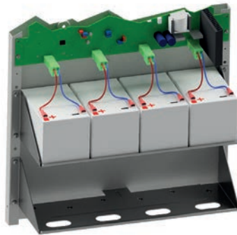
Abb. 11: Batterieaufbau 24 Ah
