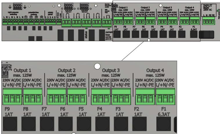
Abb. 20: Anschluss Endstromkreise
