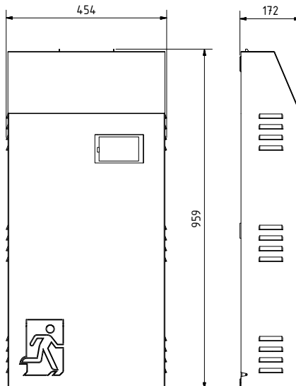
Abb. 5: Maßzeichnung LPS 230-500-M
