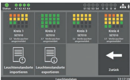
Abb. 94: Maske „Leuchten Daten – Leuchtenstandorte“
