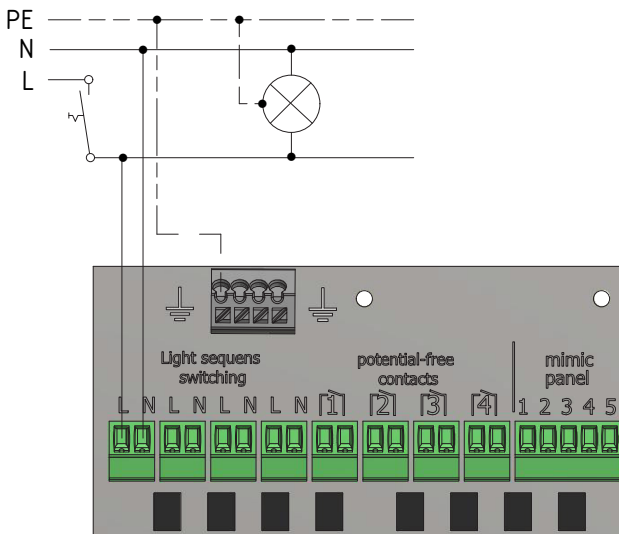
Abb. 28: Lichtsteuereingänge
